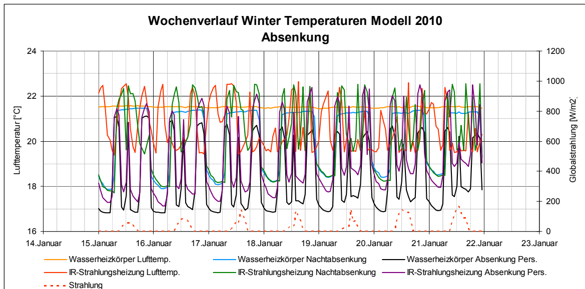
Abbildung 17 Temperaturverlauf Winterwoche, Modul Absenkung, Modell 2010
