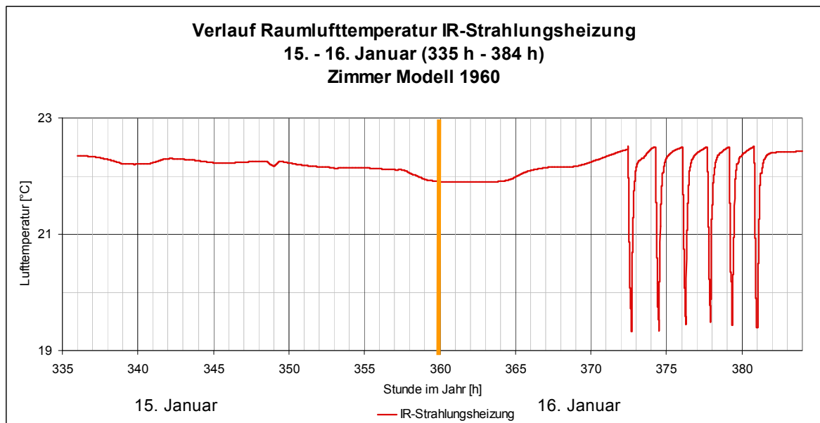
Abbildung 24 Raumtemperatur bei IR-Strahlungsheizung, 15. und 16. Januar, Modell 1960
