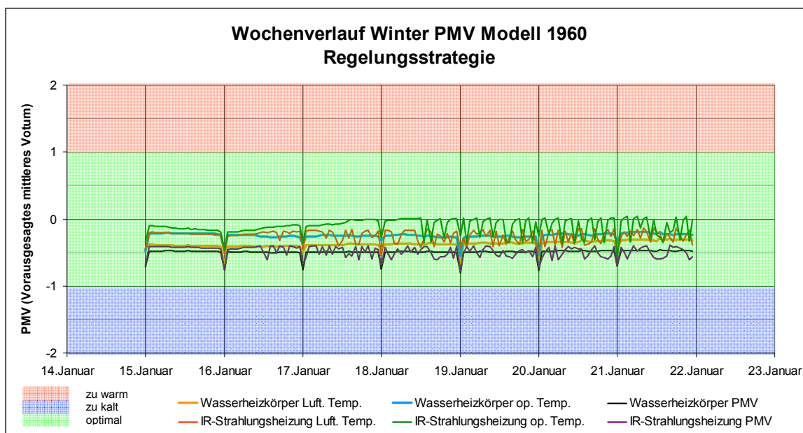
Abbildung 10 Wochenverlauf Winter, PMV-Werte, Modul Regelungsstrategie, Modell 1960
