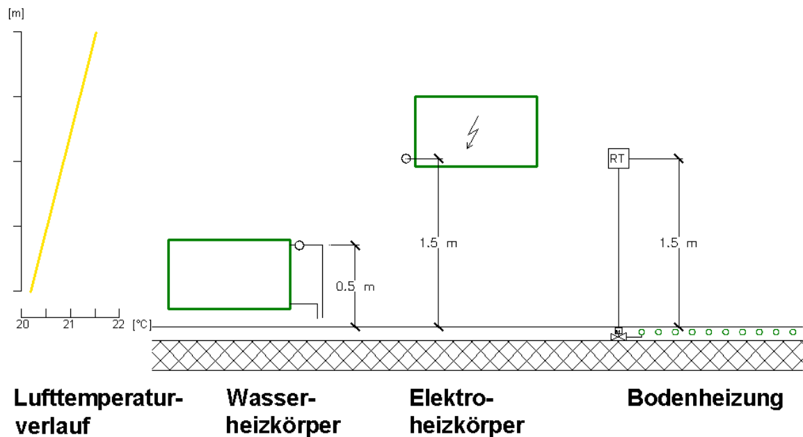
Abbildung 27 Positionierung Fühler
